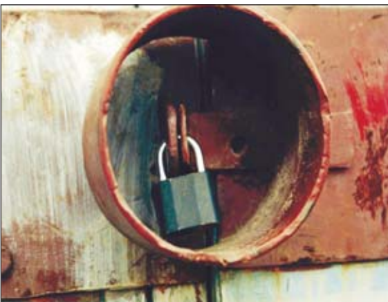
Ośłona w kształcie pierścienia zmniejsza możliwość pokonania kłódki przez jej ukrećczenie lub rozbięcie
